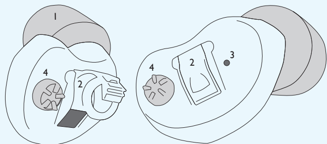
1. Gommino | 2. Sportello pila | 3. Microfono | 4. Potenziometro 1. Foam pad | 2. Battery holder tab | 3. Microphone | 4. Potentiometer
